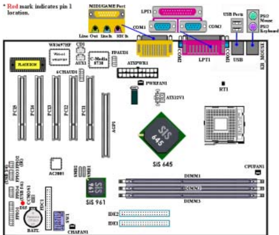
圖 1-1. SD7-533 主機板重要零件位置圖
