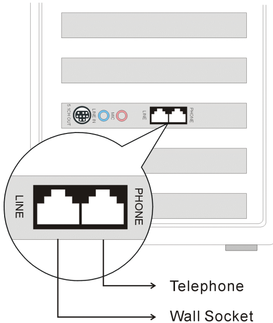
圖 2-4. 先連接牆壁上的電話插座到「LINE」輸入孔，然後連接「PHONE」輸出孔到電話機。
