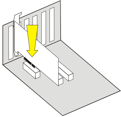
圖 2-3. 安裝 AC10 到 CNR 擴充槽
