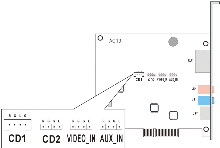
圖 2-2. CD1 ~ AUX_IN 接頭的接腳定義
