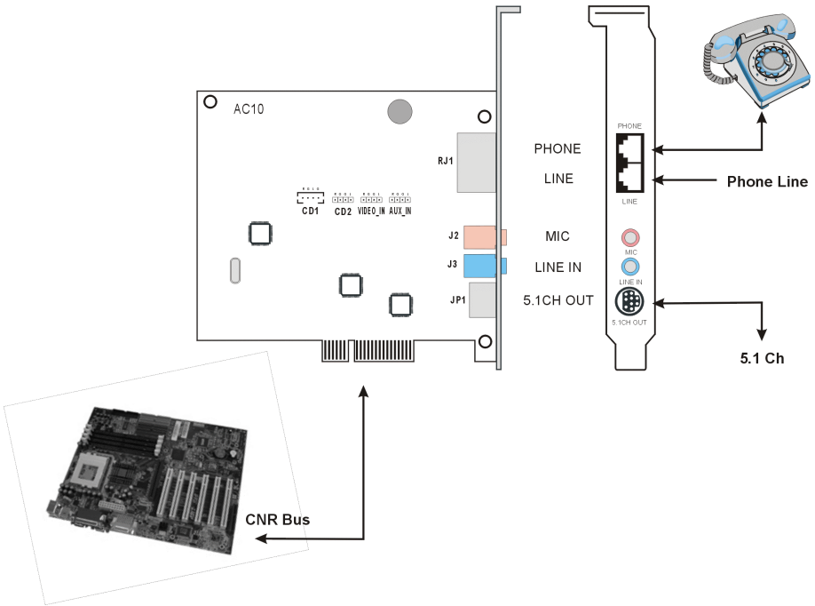
圖 2-1. AC10 CNR 卡配置圖
