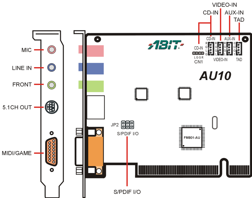
圖 2-1. ABIT Home Theater AU10 音效卡的連接示意圖
