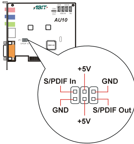
圖 2-2. S/PDIF I/O 端子的接腳定義
